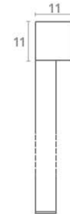
CLICK ZIP 11 larghezza / width fino a / up to cm 400 altezza / height fino a / up to cm 380
